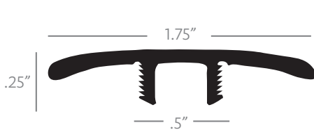
T-MOLD
