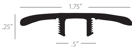
T-MOLD
