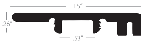
END CAP
