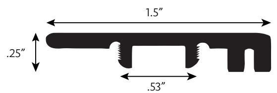
END CAP
