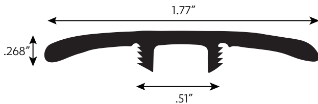
T-MOLD
