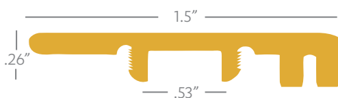
END CAP
